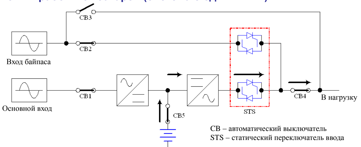
Рис.2-2 Режим работы от батареи (один ИБП)
